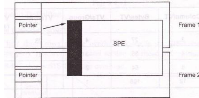
Fig. 8.4.10 SPE in STS-1 frame
