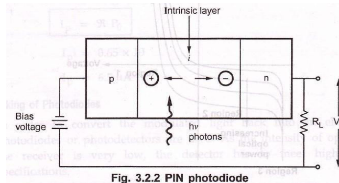
Fig. 3.2.2 PIN photodiode
