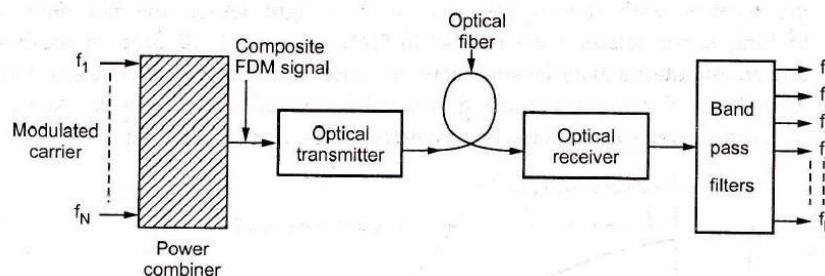
Fig. 6.1.4 Multichannel AM SCSVMV
